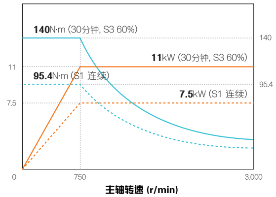
铣削刀座 3,000 rpm 功率(kW) 扭矩(N·m)
