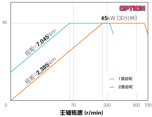
L700L系列 (大孔径) 700 rpm 功率(kW)
