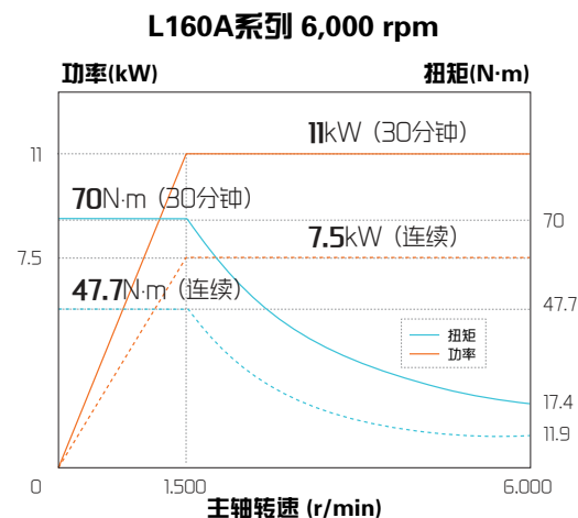
主轴电机功率/扭矩图 (现代威亚 FANUC i 系列)
